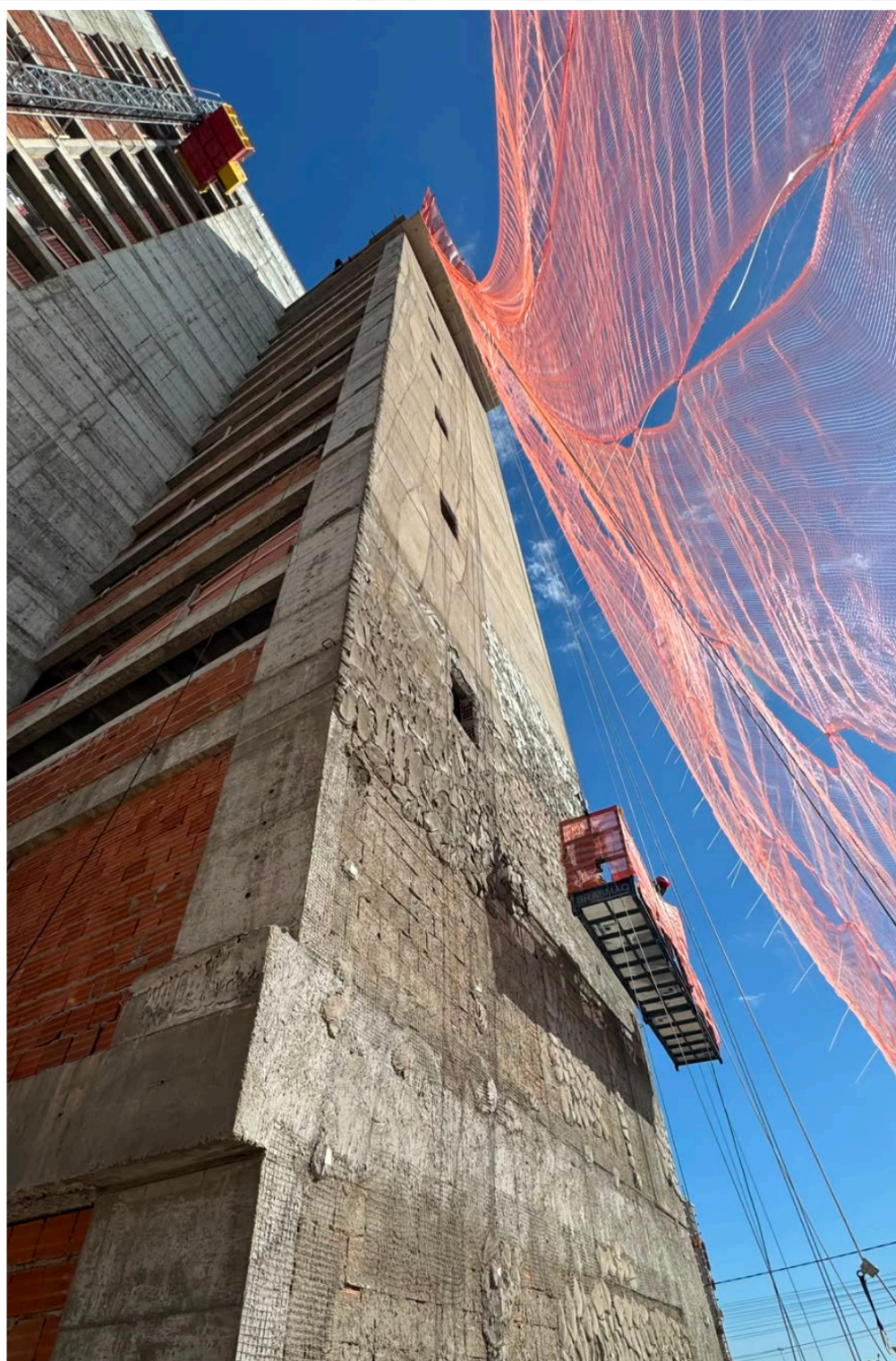
Reboco Externo - Balancim
