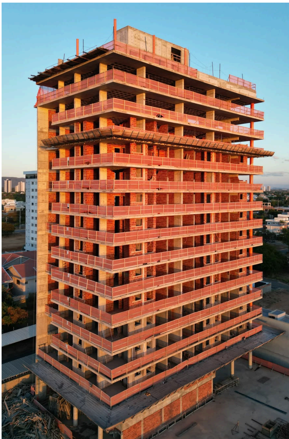
Vista Externa - Frontal/Lateral
